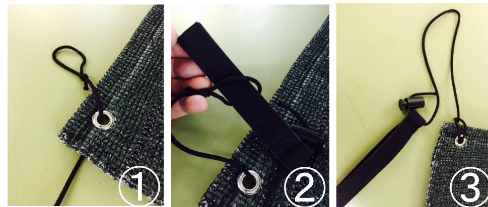
(上写真) 面ファスナー部分はBack to Back MOLDタイプ。本仕様では2つ折りで溶着し、輪っかが作られているのがミソ。ハトメに輪っかを通し、その輪っかに面ファスナー部材を通すだけの3ステップでネットへの固定は完了。あとは張るだけだ。
